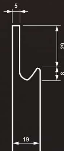
Схема загального торцевого профіля усіх трьох видів ручьок (С, V і N)
